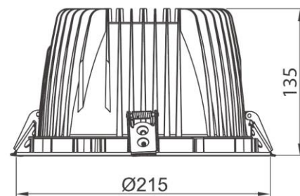
Габаритные размеры
