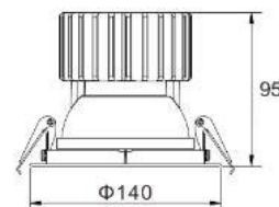
Габаритные размеры
